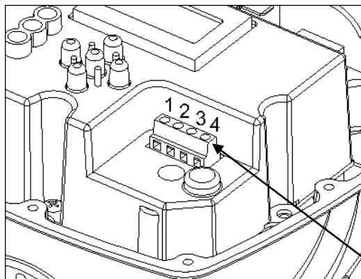
KONEKTOR POMOCNÝCH KONTAKTŮ
